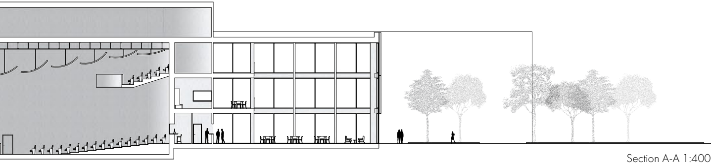
Section A-A 1:400
