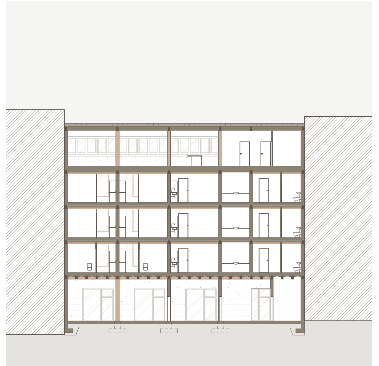
Longitudinal section 1:200
