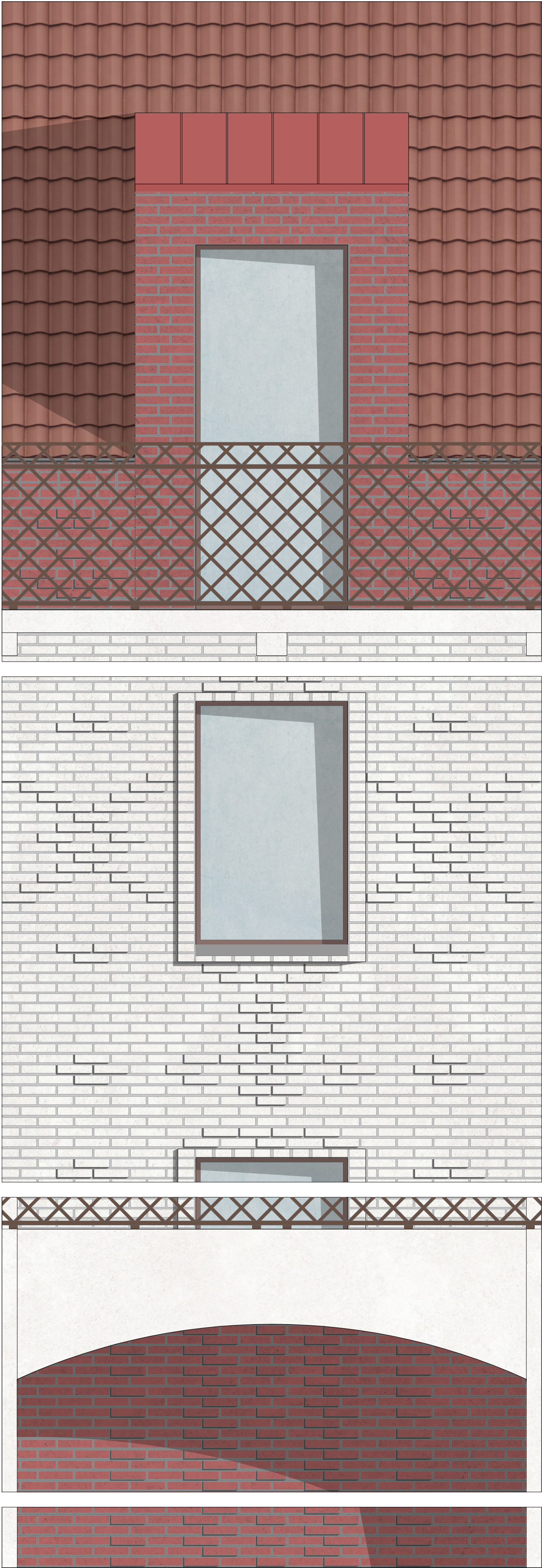
FASADUTSNITT 1:20
