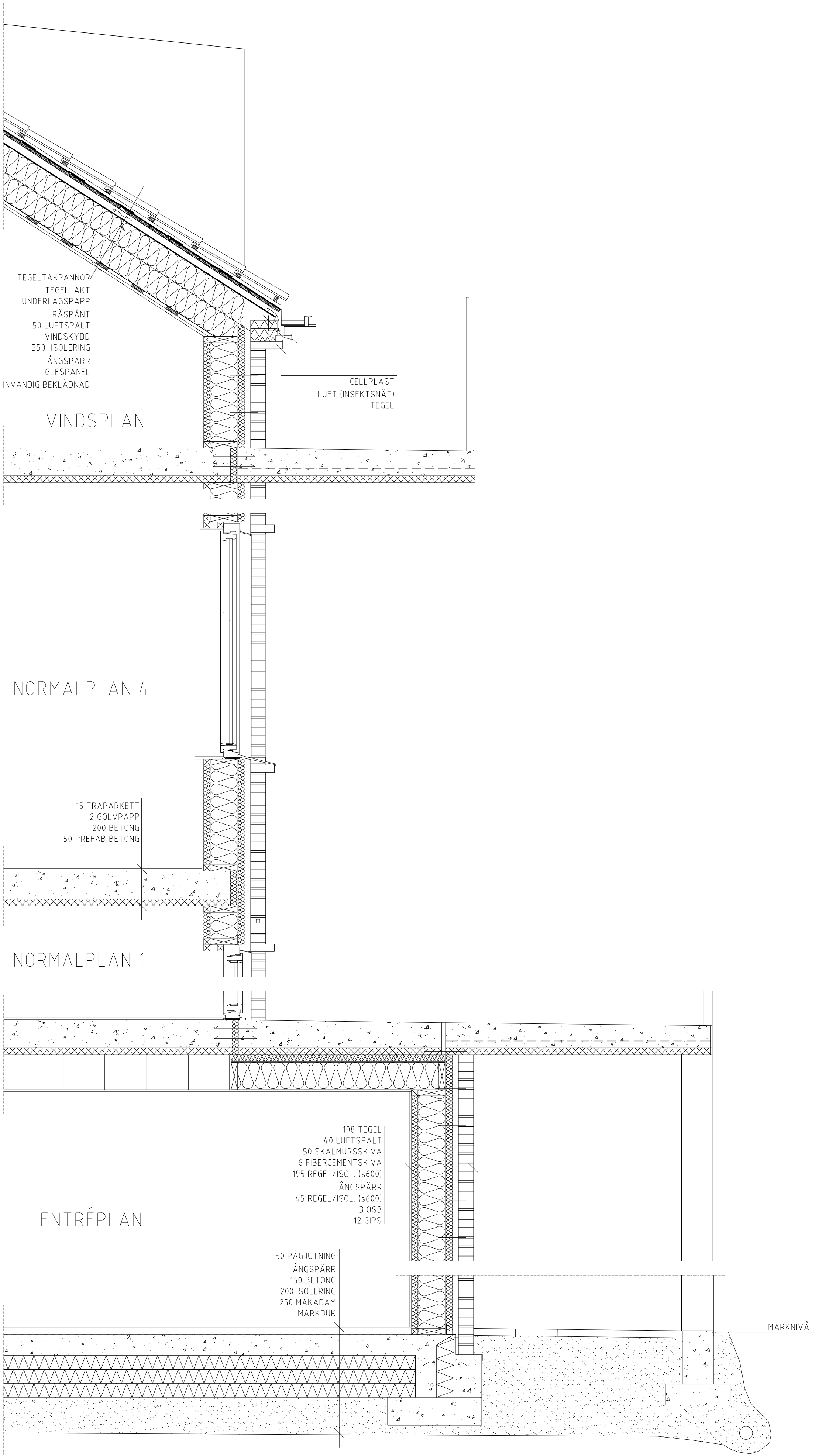
PRINCIPSEKTION 1:20
