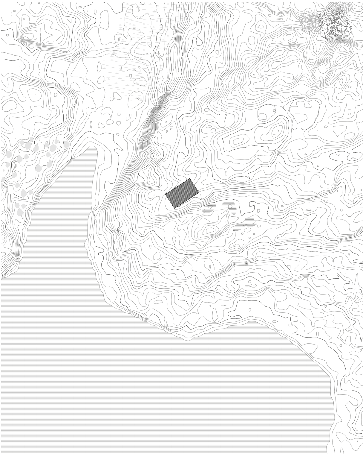
Site plan 1:400
