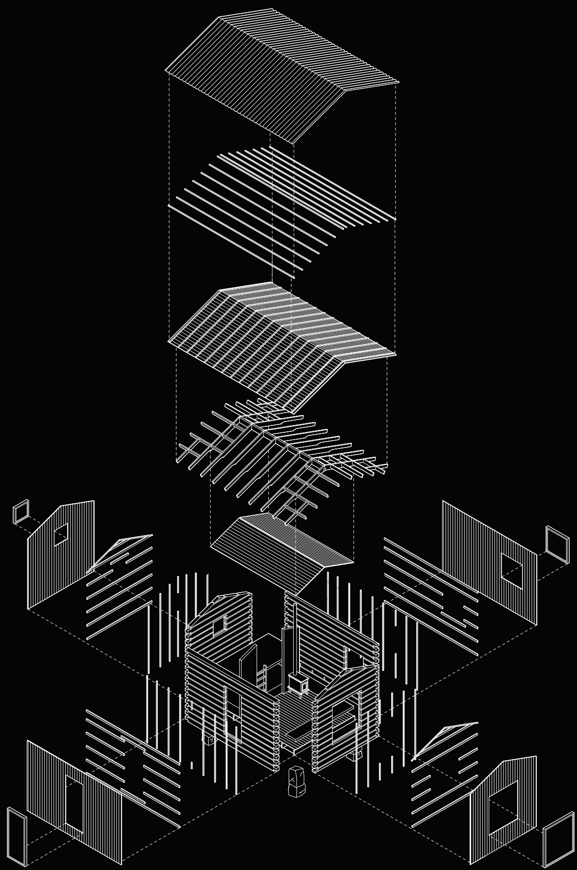
Axonometric Log Timber
