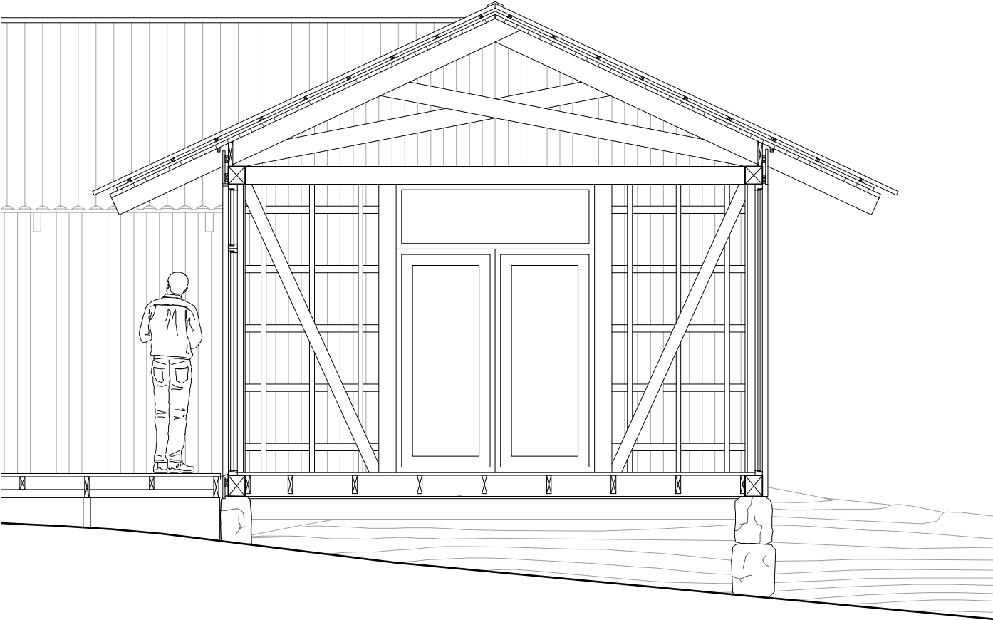
Section A-A
