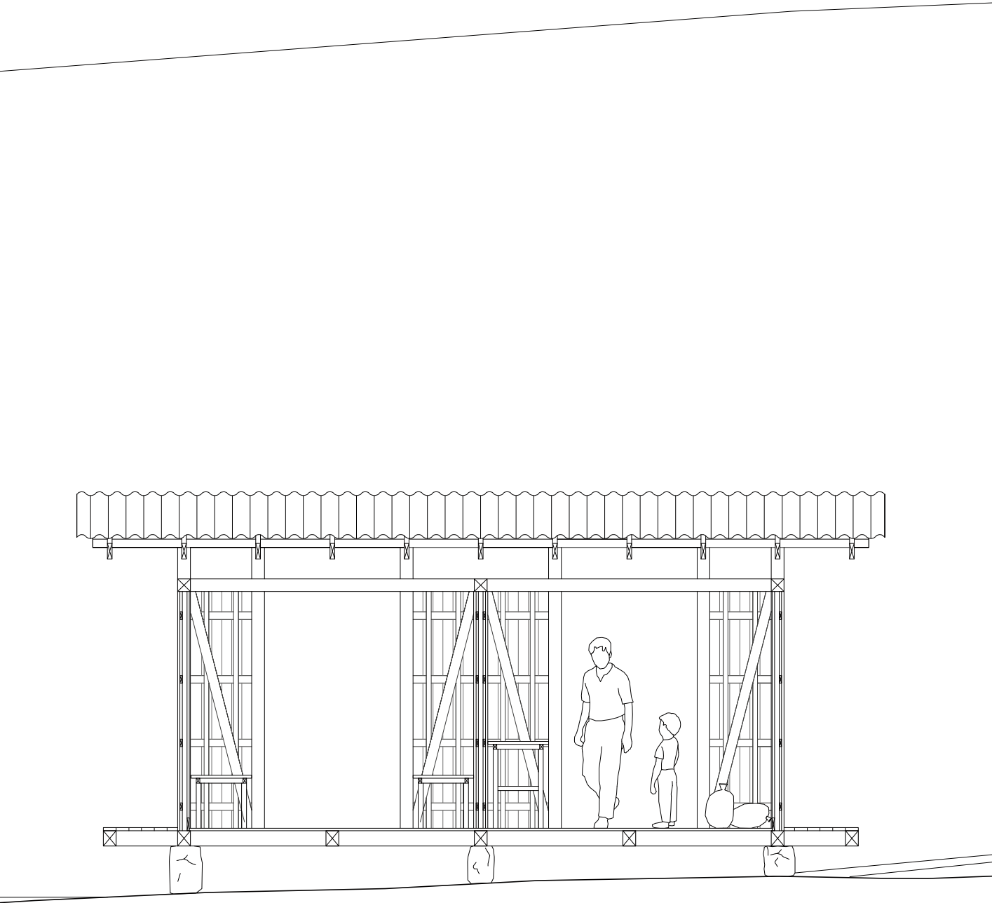
Section A-A 1:50
