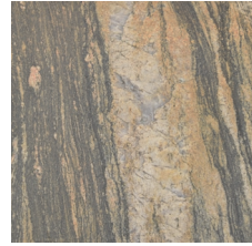
Migmatit
