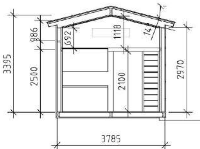
Sektion, alternativ 3
