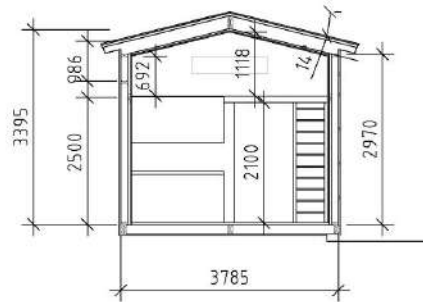
Sektion
