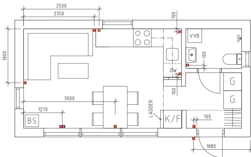
Installationsritning - Plan 1 Eluttag och Telekomuttag
