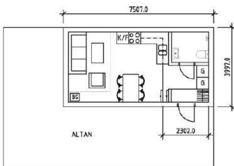
Stomritning, alternativ 3
