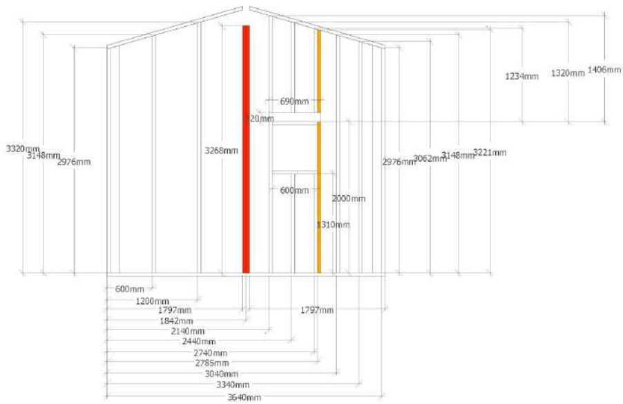
Vägg 3 - mot öster
