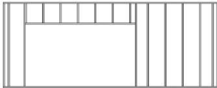
Stomritning, alternativ 3
