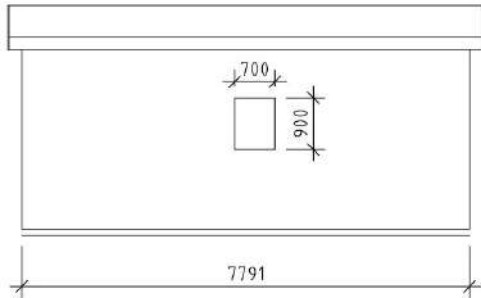
Fasad - 14 graders taklutning
