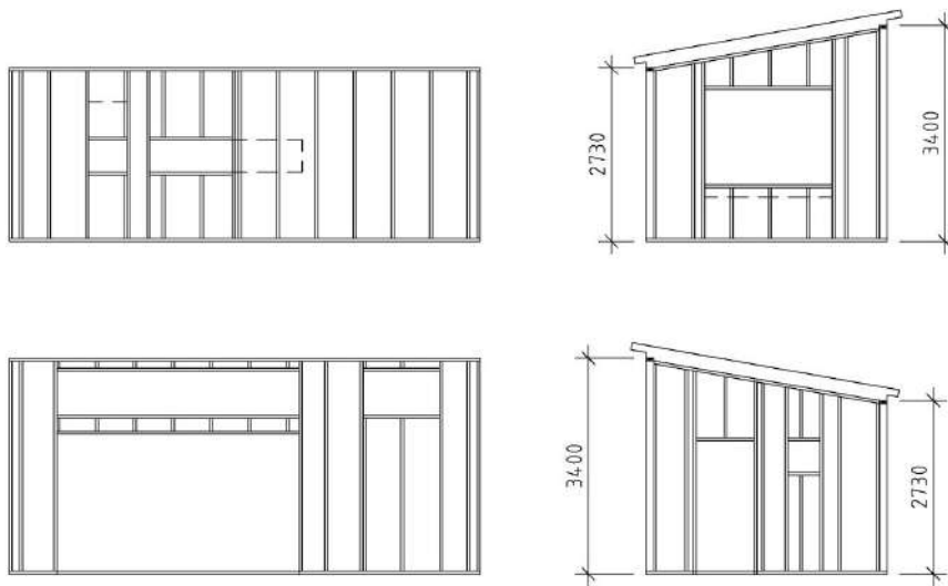
Stomritning, alternativ 1
