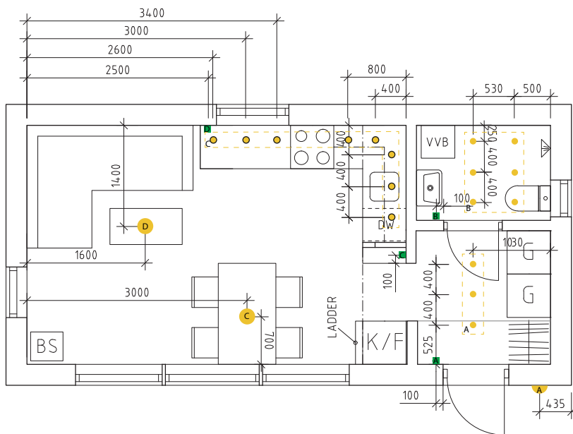
Installationsritning - Plan 1 Lampor och strömbrytare
