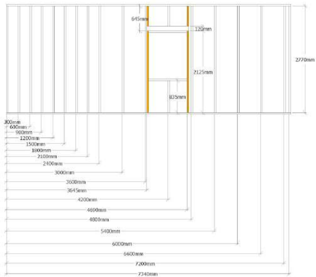
Vägg 2 - mot norr
