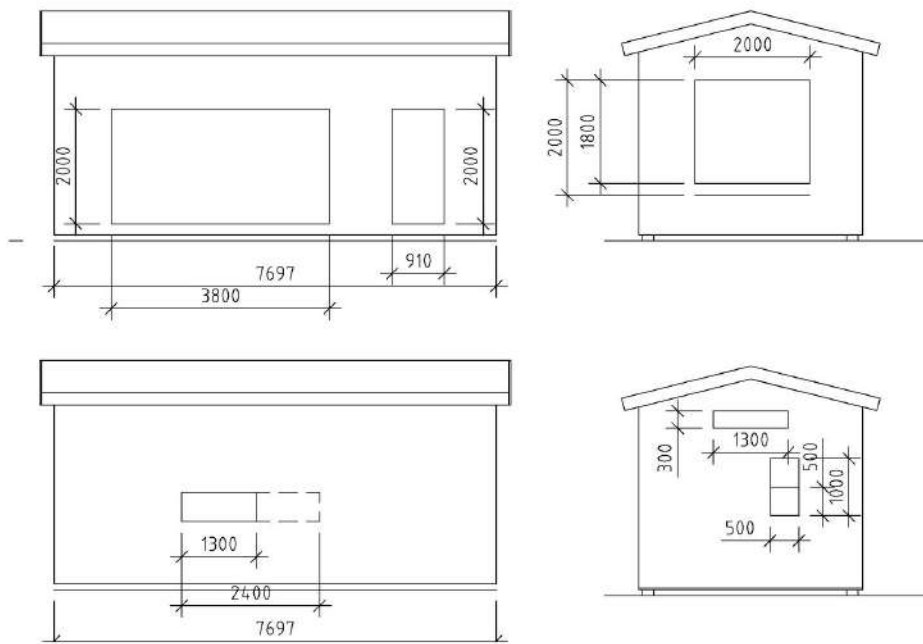
Fasader, öppningsmått (intervallmått)
