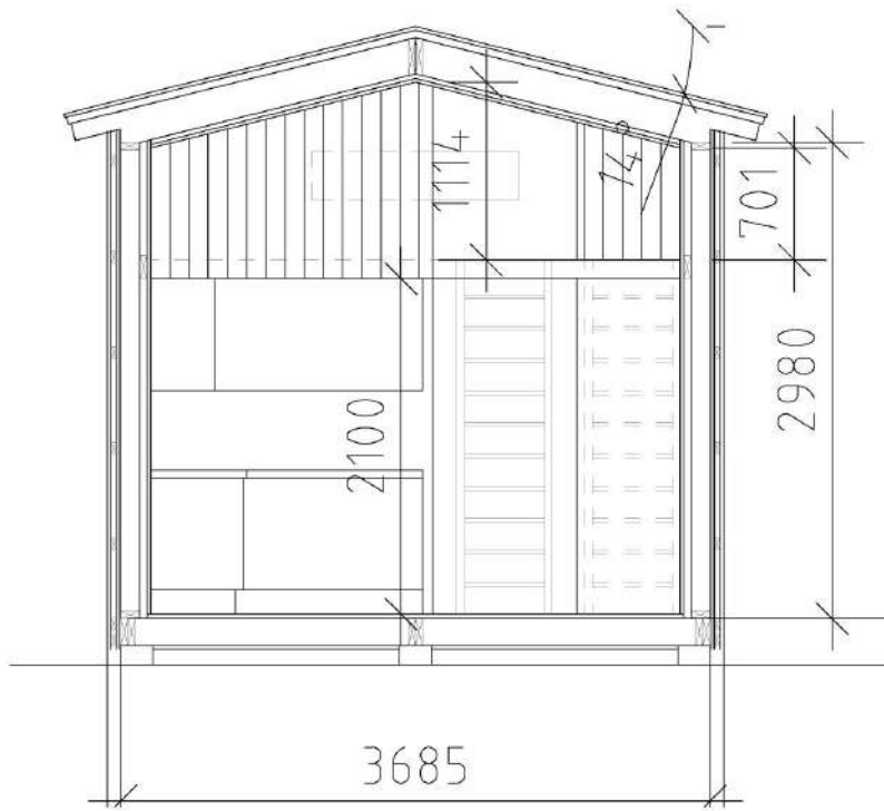
Sektion, 14 graders taklutning
