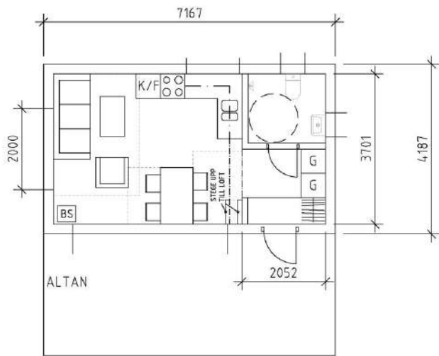
Planlösning, tillgänglig
