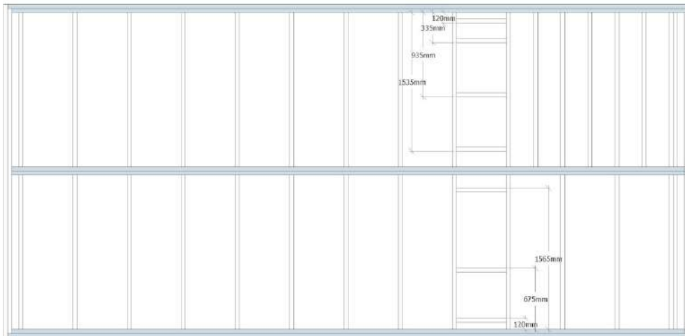
Bjälklag - måttsatt
