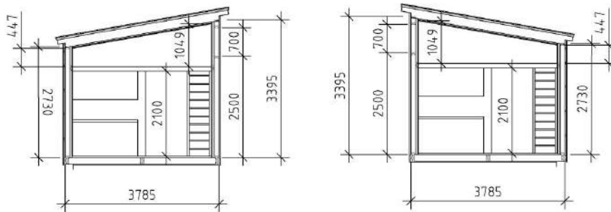
Sektion, alternativ 1
