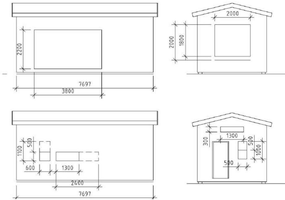
Fasad, alternativ 3
