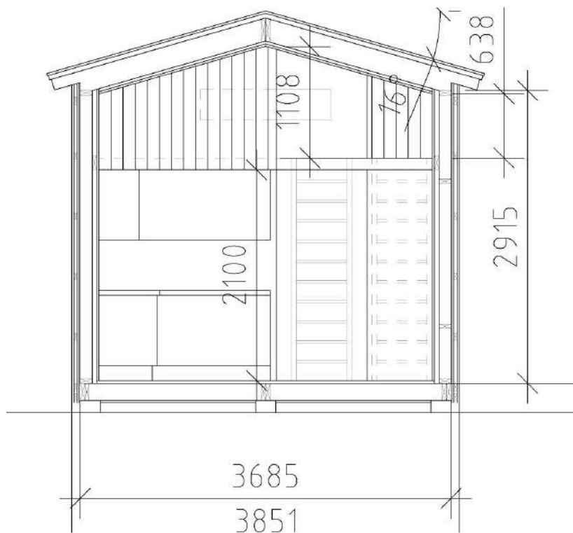
Sektion - 16 graders taklutning
