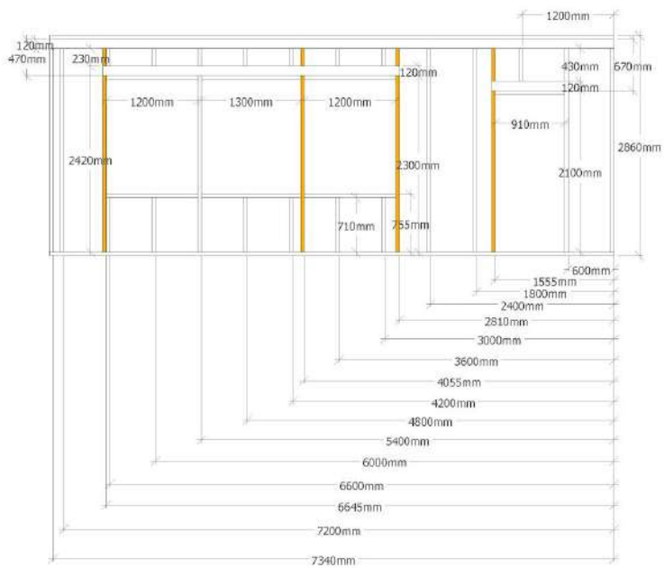
Vägg 1 - mot söder
