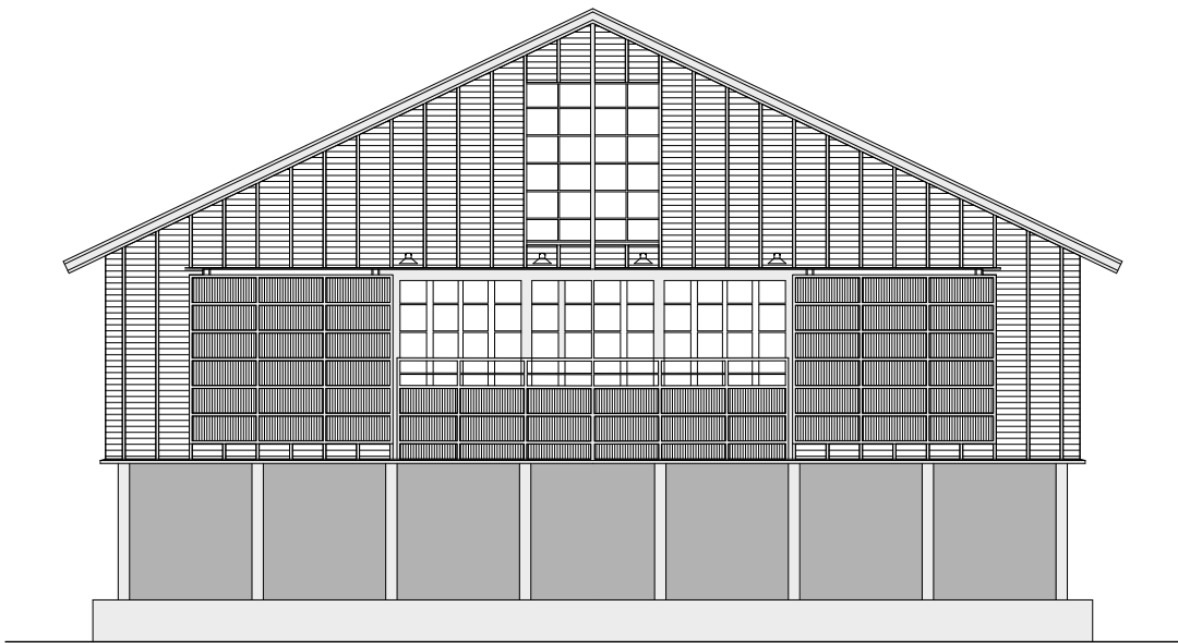
Fig. 34. Drawing of Sågen
