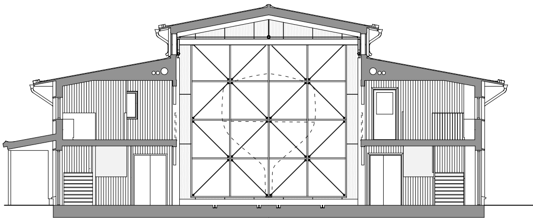
Fig. 73. Section B-B
