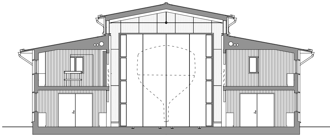
Fig. 71. Section A-A
