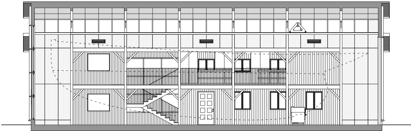
Fig. 74. Section D-D
