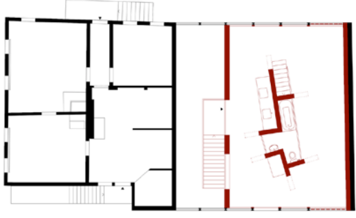
Fig. 05 Freiluft barn, plan
