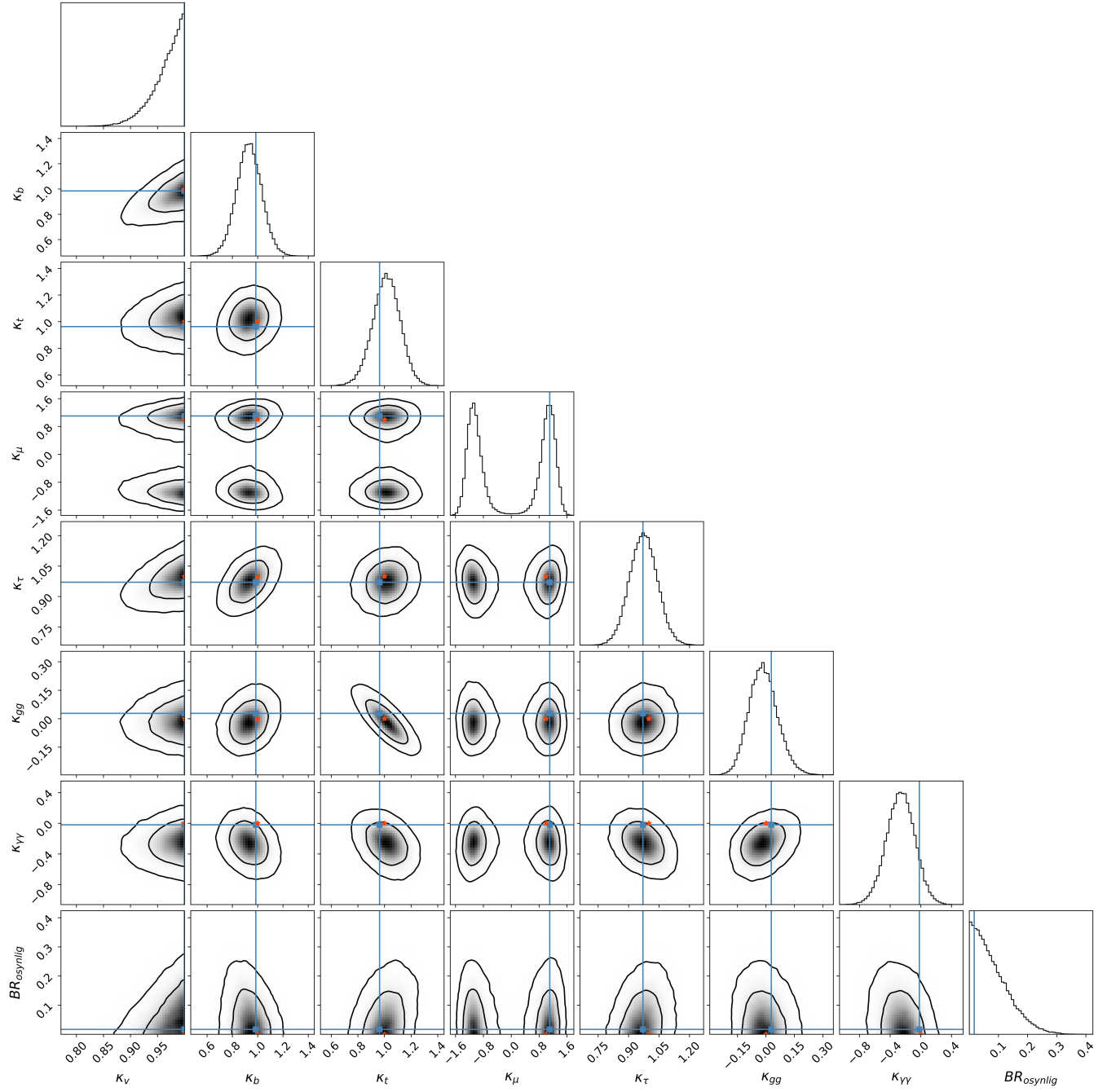
Figur 6.7: A posteriorifördelningar för modelloberoende analys med åtta parametrar, där \kappa_W = \kappa_Z = \kappa_V och BR_{0synlig} \neq 0 . Den heldragna linjen indikerar bästa anpassnings-värdet. I konturdiagrammen indikerar mörkare områden mer sannolikhet. Avgränsande linjer är 68 % och 95 % konfidensområden. Stjärnan indikerar SM-värdet.
