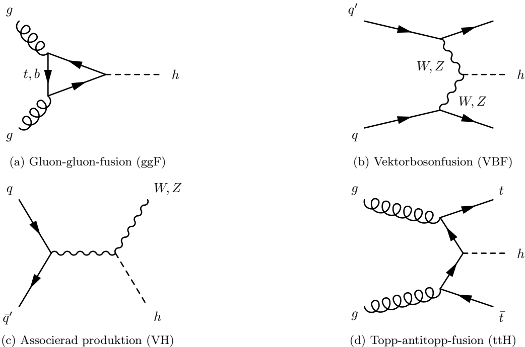
Figur 3.2: Representativa feynmandiagram för higgspartiklens produktionskanaler i LHC. Fler feynmandiagram förekommer för dessa processer. Kvarkar är betecknade q och q' . Diagrammen är anpassade från [10].
