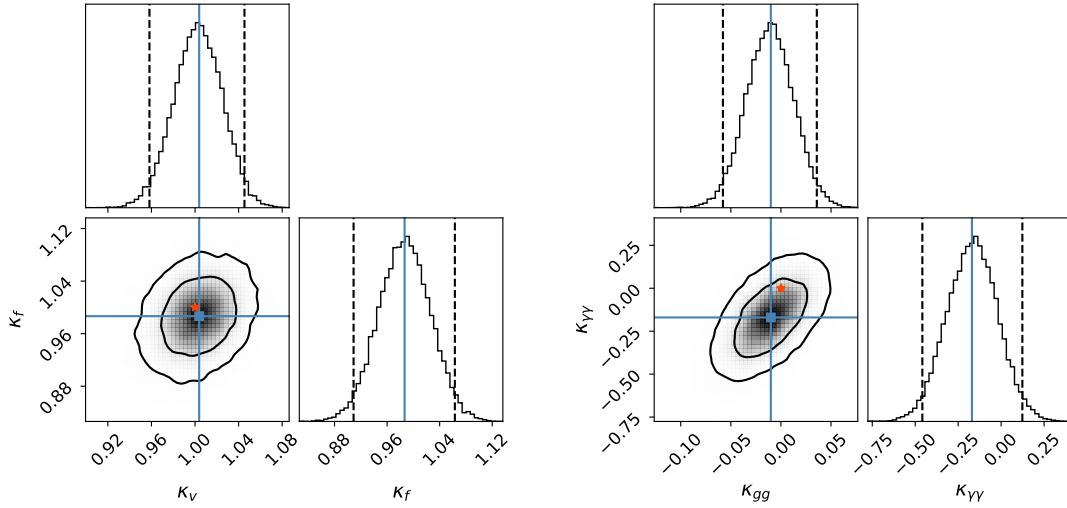
(a) Varierande parametrar \kappa_V och \kappa_f .
