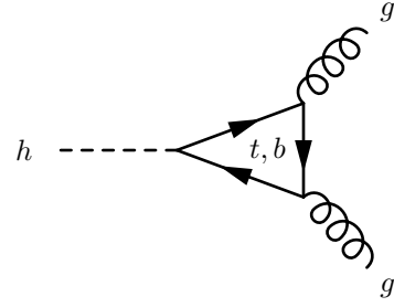
(b) Sönderfall till två gluoner hgg .
