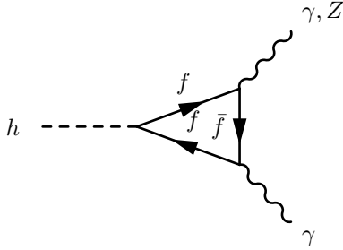
(c) Sönderfall till två fotoner h\gamma\gamma eller foton och Z-boson hZ\gamma .
