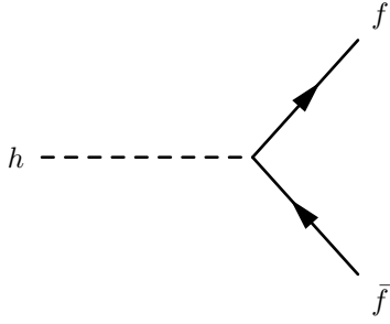
(a) Sönderfall till fermioner hf\bar{f} där f = \mu, \tau, b, c .
