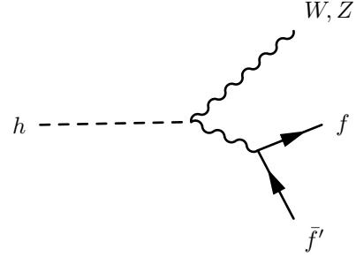
(d) Sönderfall till vektorbosoner och leptoner hV .
