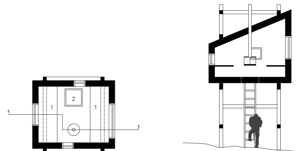
Plan 1:100
