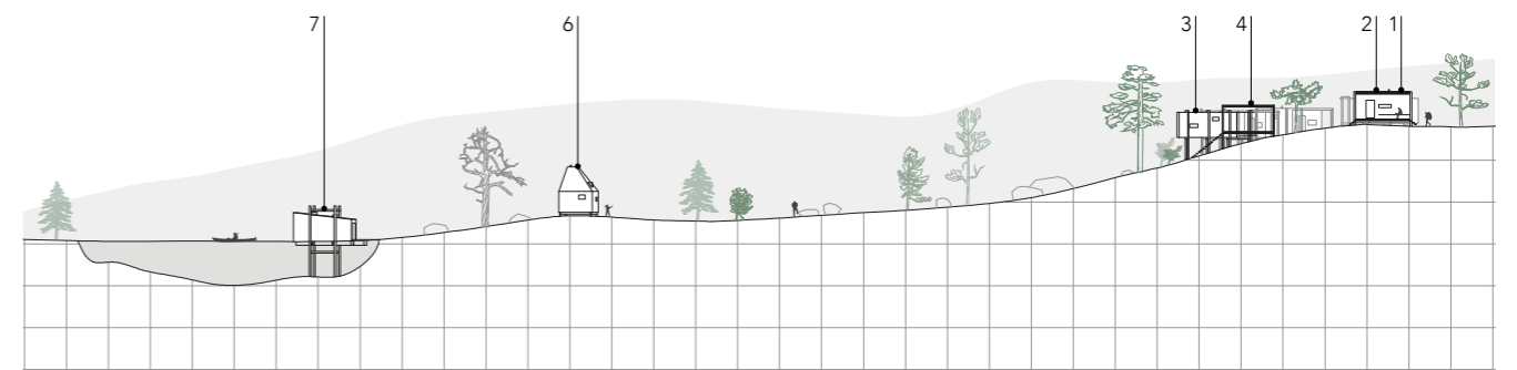
Site section 1:1000
