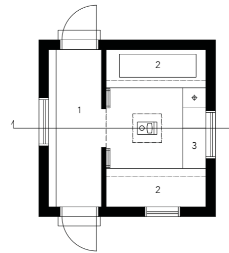
Plan 1:100
