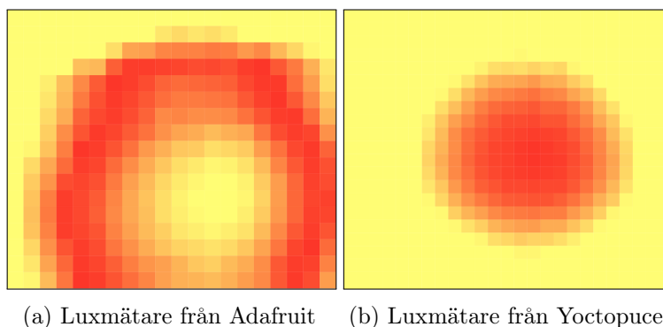
Figur 4.5: Uppmätt ljusstyrka
