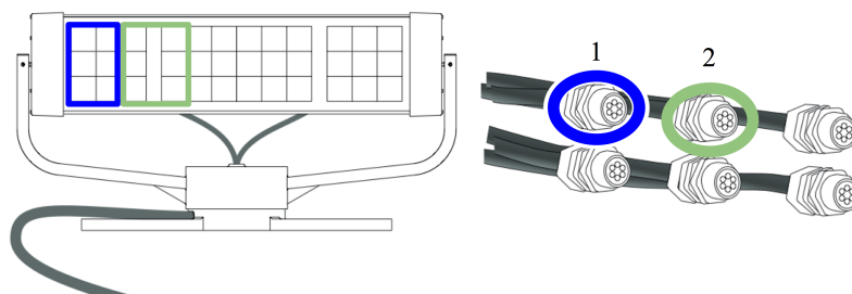
Figur 4.3: Översikt av rundgångskoppling
